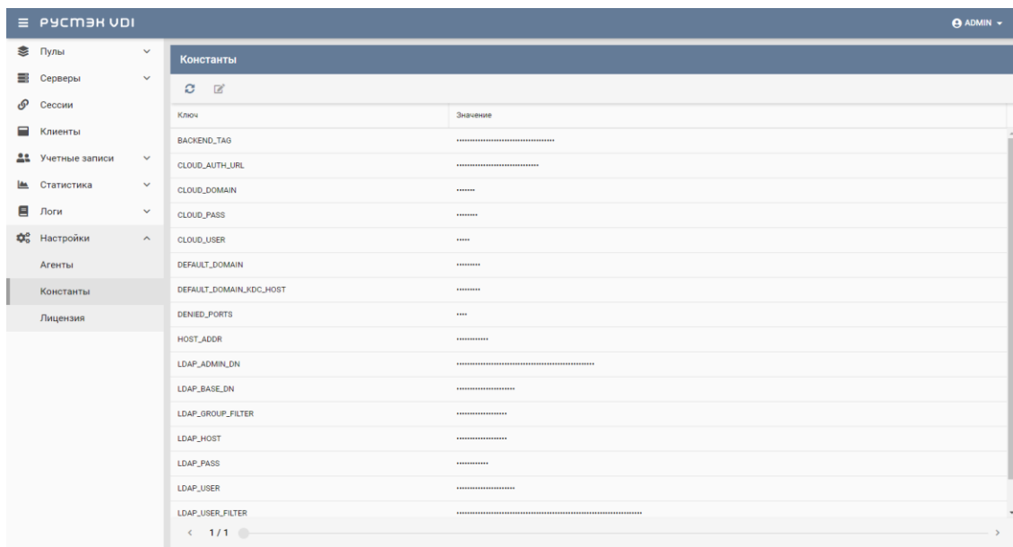
Рисунок 27 – Раздел меню Настройка – Константы
