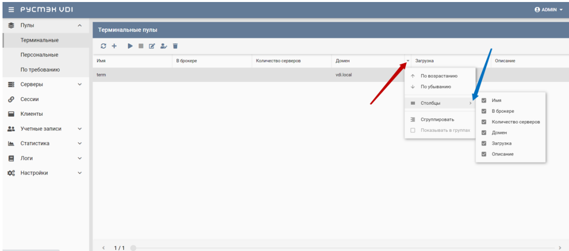
Рисунок 4 – Выбор столбцов
